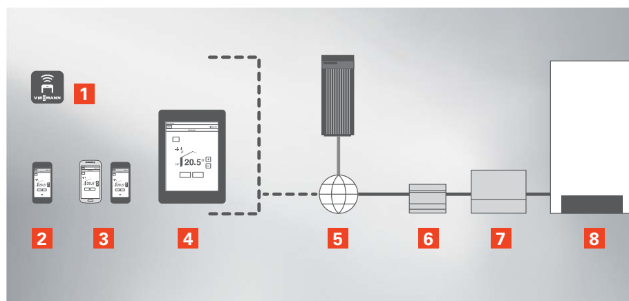
Schemat instalacji modułu Vitocom 100 LAN
